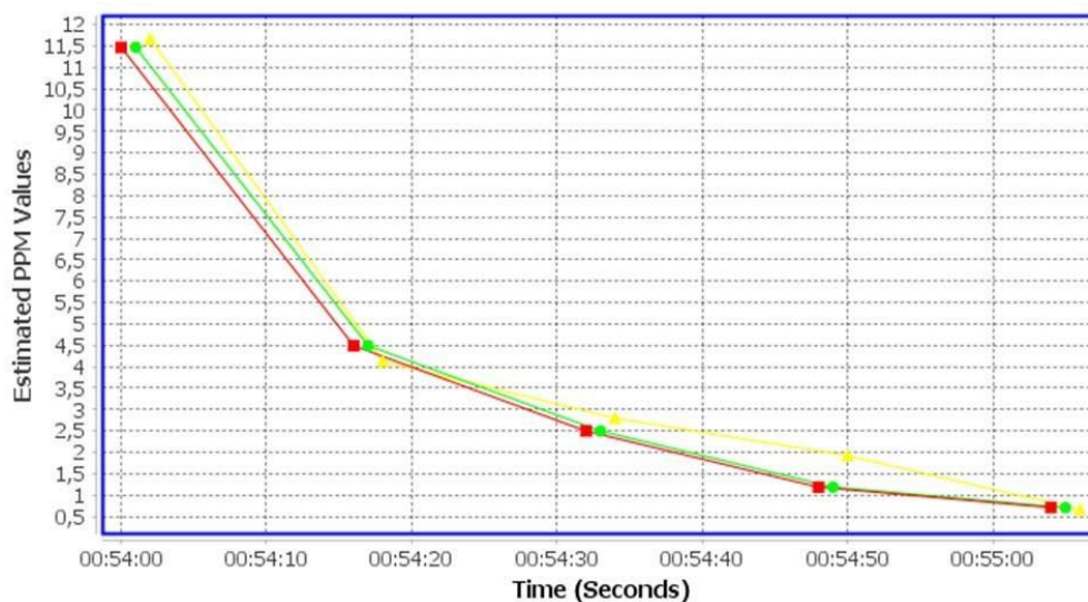
Fig. 4 E3 Traffic estimation result
