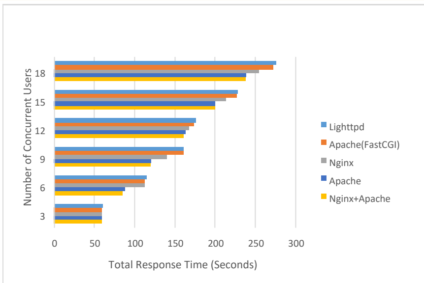
Fig. 6 HADAS: PHP web service graphs
